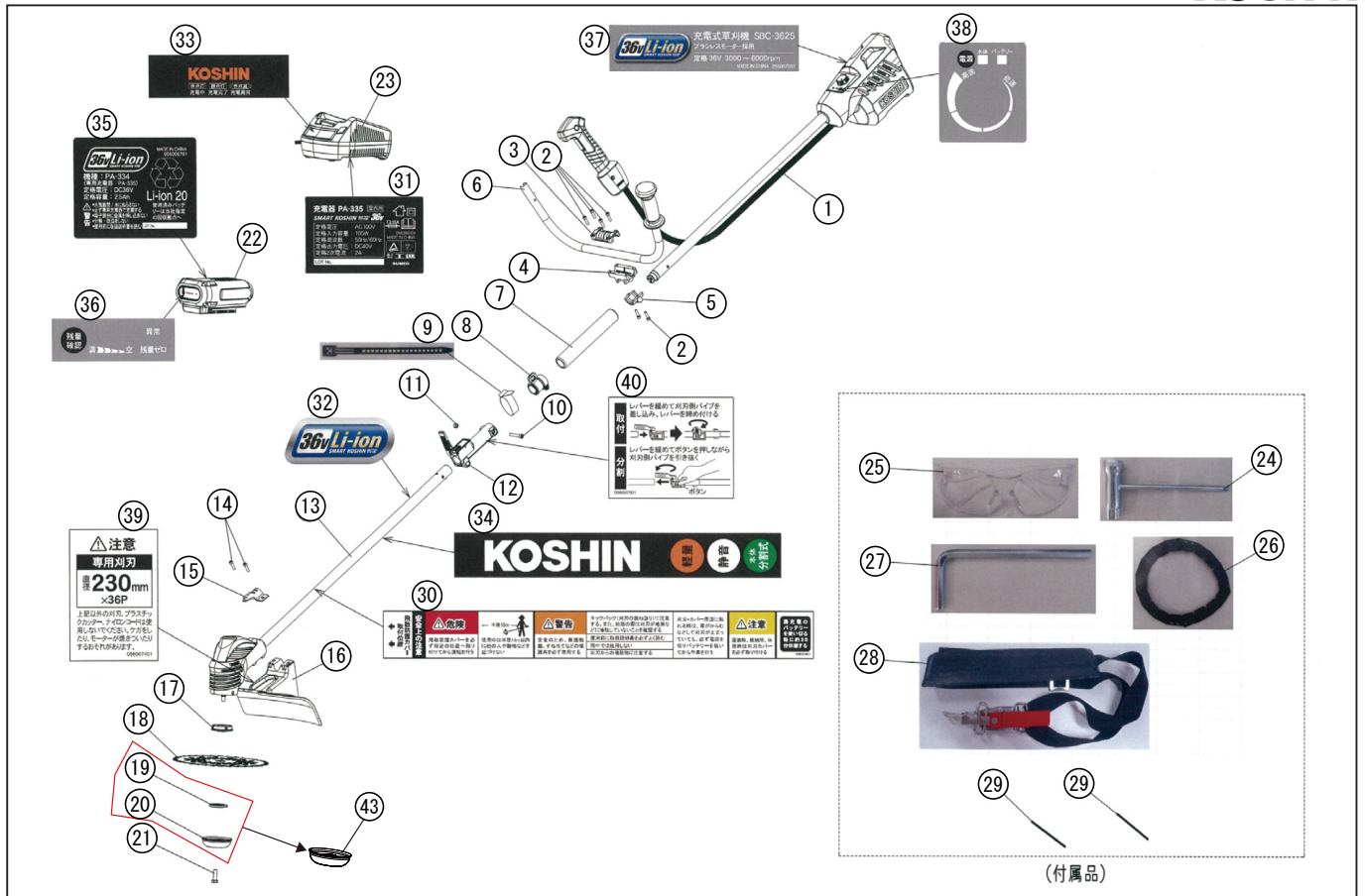
型式名 SBC-3625-AAA-0 (056851302)
