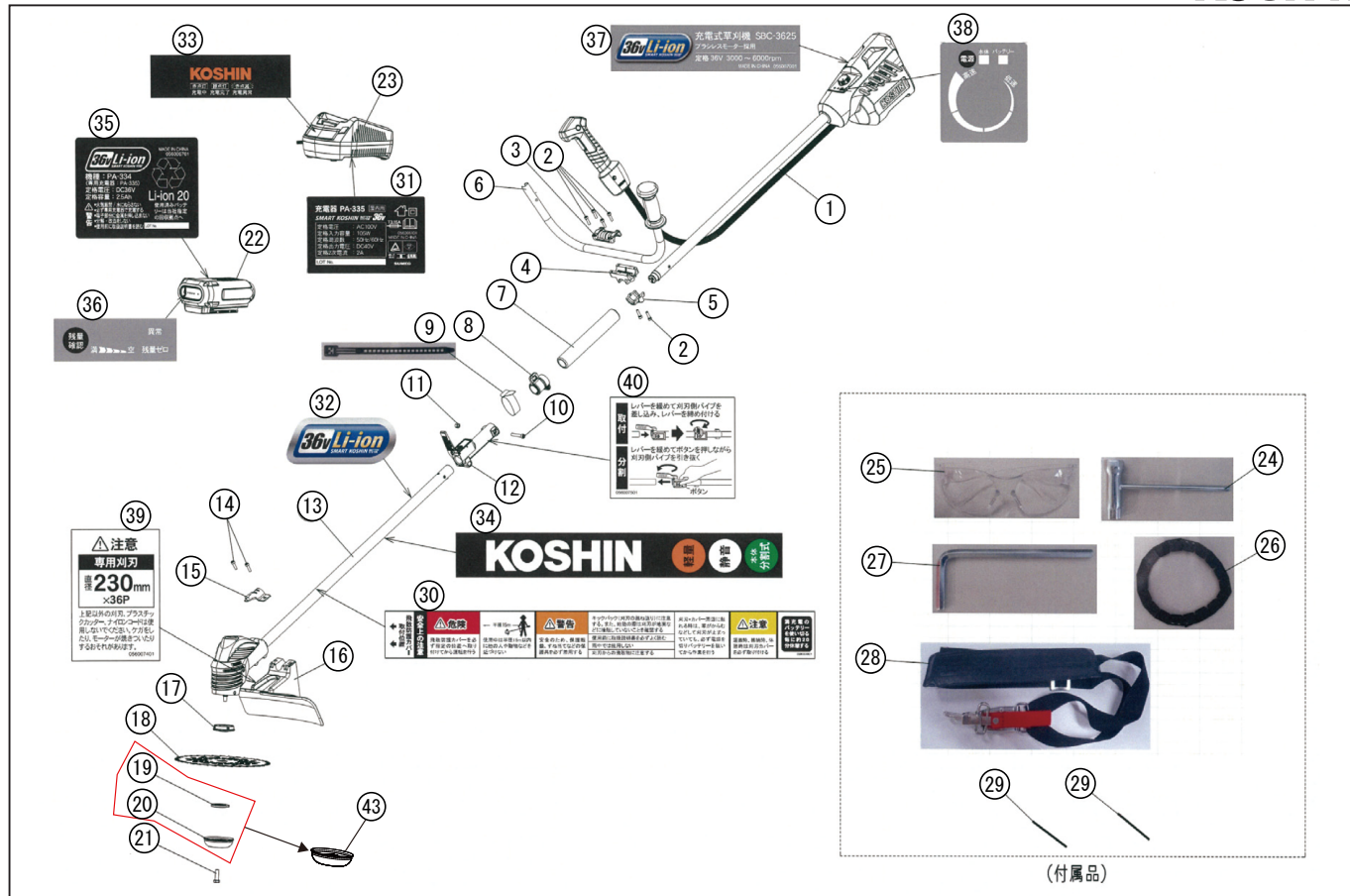
型式名 SBC-3625-AAA-0 (056851302)
